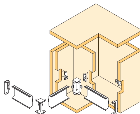
Profil de tiroir horizontal "C".
