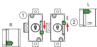
commutation du sens de verrouillage
