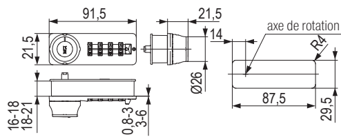
schéma de l'ouverture dans le panneau 16–21 mm
