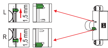
activation du blocage de clé (la clé ne peut pas être retirée de la serrure déverrouillée)
