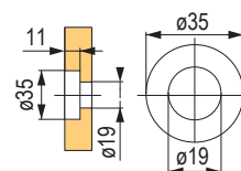
perçage dans le bois
