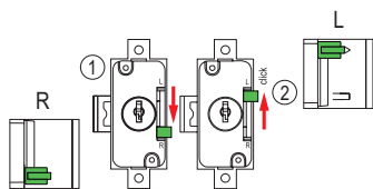
commutation du sens de verrouillage
