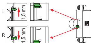
activation du blocage de clé (la clé ne peut pas être retirée d'une serrure déverrouillée)
